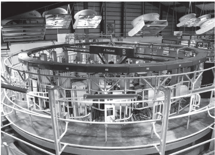
ロータリー型自動搾乳ロボット（24頭搾乳可能）
